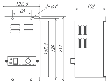
トランスボックス (共通)
