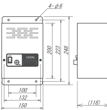
トランスボックス FT-C402
