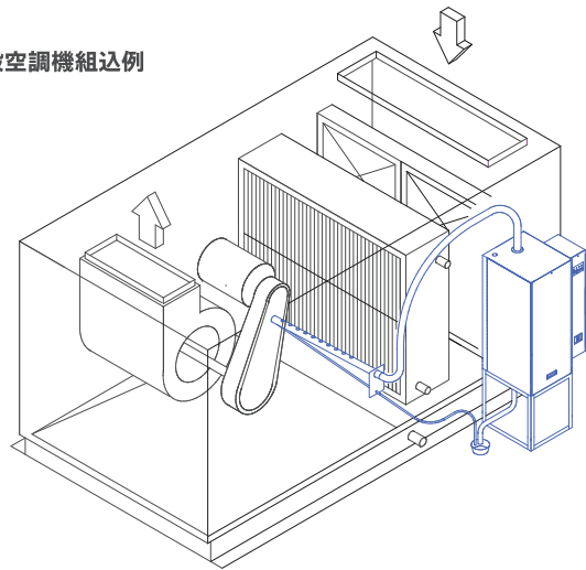
ダクト組込例
