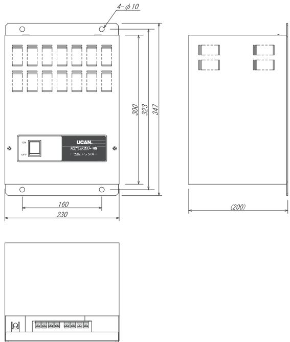
トランスボックス FT-F165~245用
