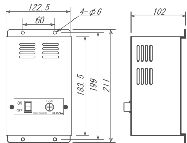
トランスボックス FT-C202
