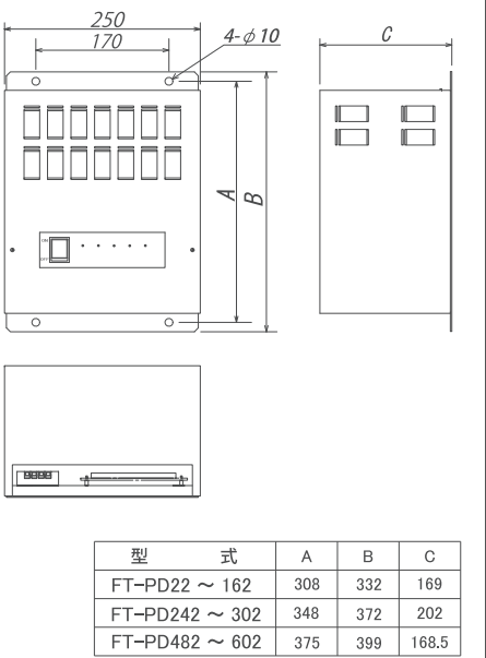
FT-PD トランスボックス
