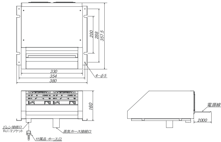
一般空調機組込例
