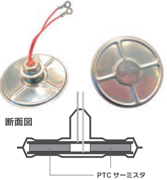
PTC水中ヒーター (型式：UCH-2100/2200)
