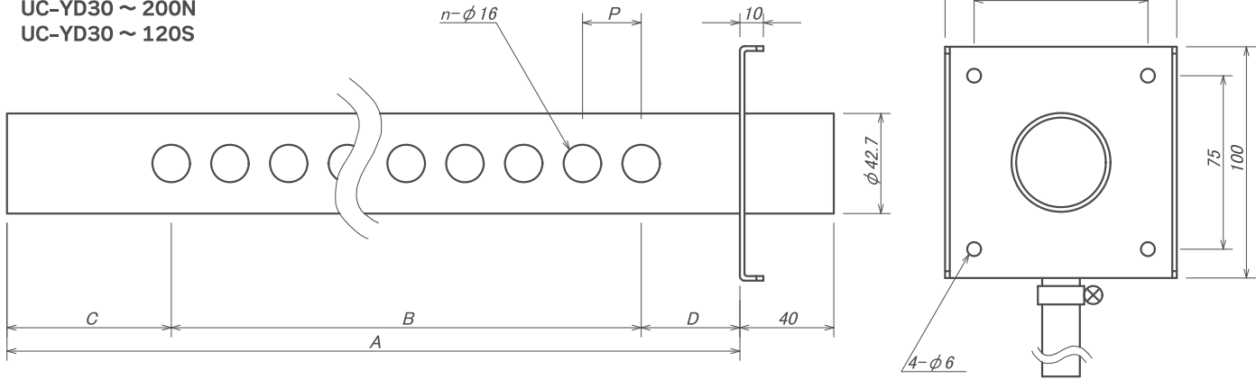
UC-YDN用蒸気ノズル対応表
