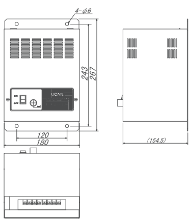
トランスボックス FT-P62 ～ 162
