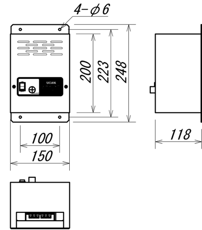
■FT-F45 トランスボックス外形寸法図
