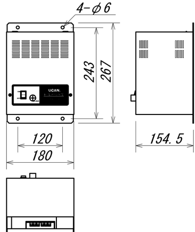
■FT-F85～125 トランスボックス外形寸法図
