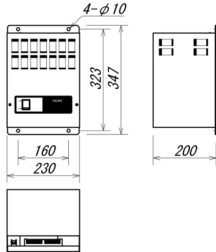
■FT-F165～245 トランスボックス外形寸法図
