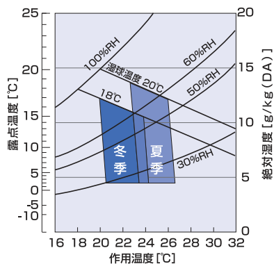
図-1 快適線図
