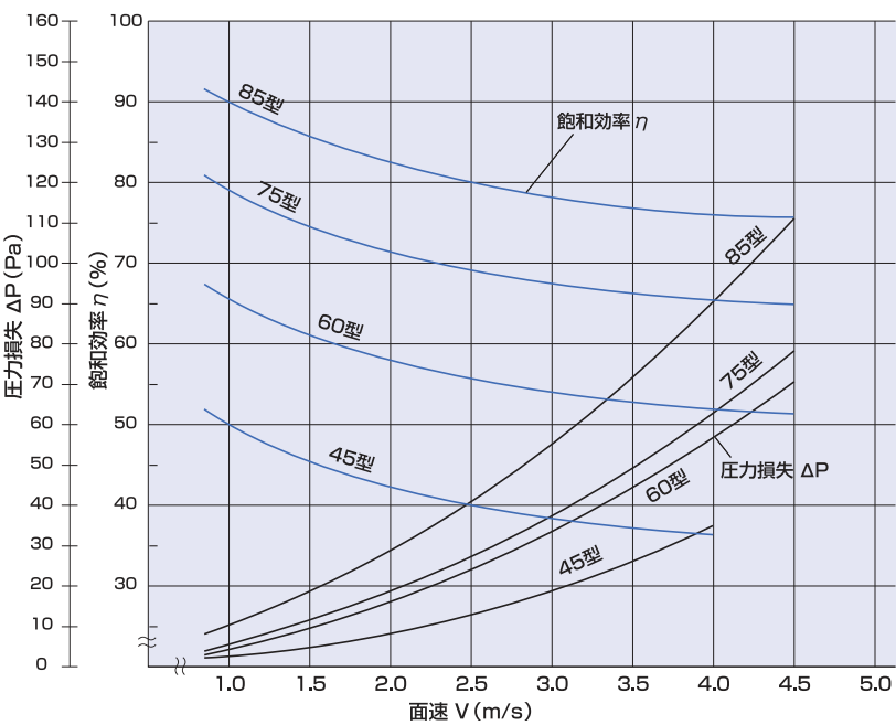
清水流下気化式加湿器「UC-EM1/EU1型」性能表
