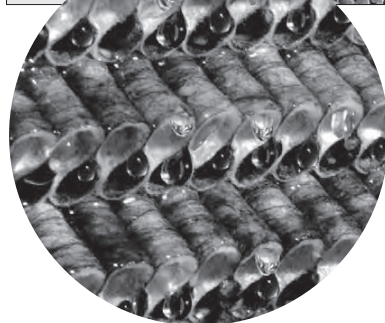
保形強度の高いハニカム積層・接着タイプ
