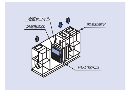
●コンパクトタイプ空調機
